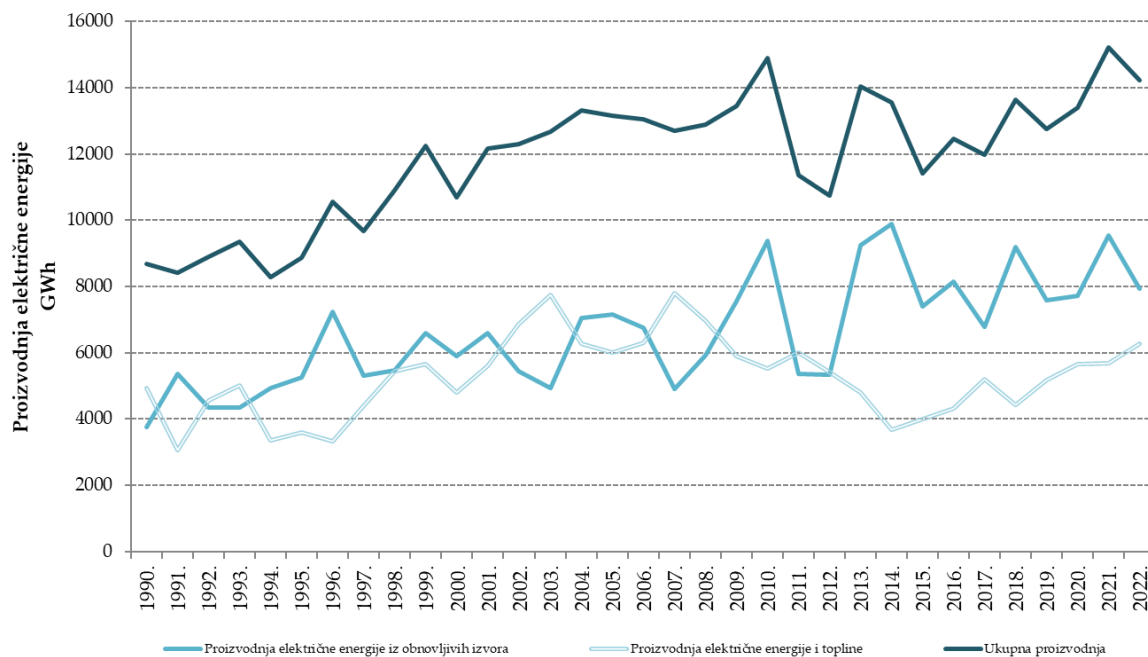
Slika 3.2-4: Proizvodnja električne energije po izvorima u razdoblju 1990. do 2022. godine
