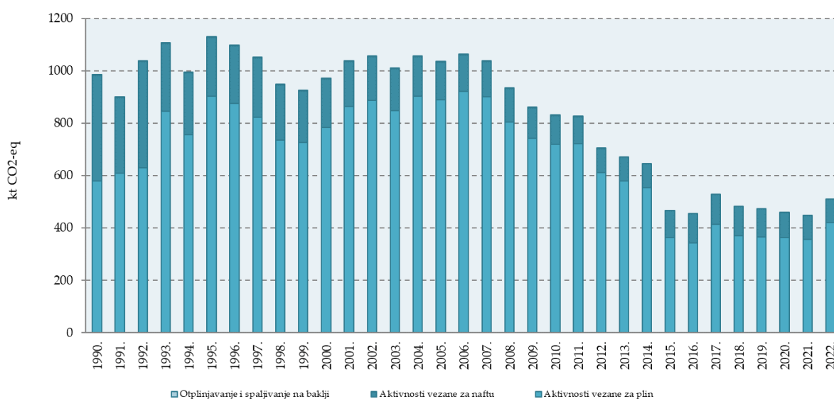
Slika 3.3-2: Fugalne emisije iz sirove nafte i prirodnog plina
