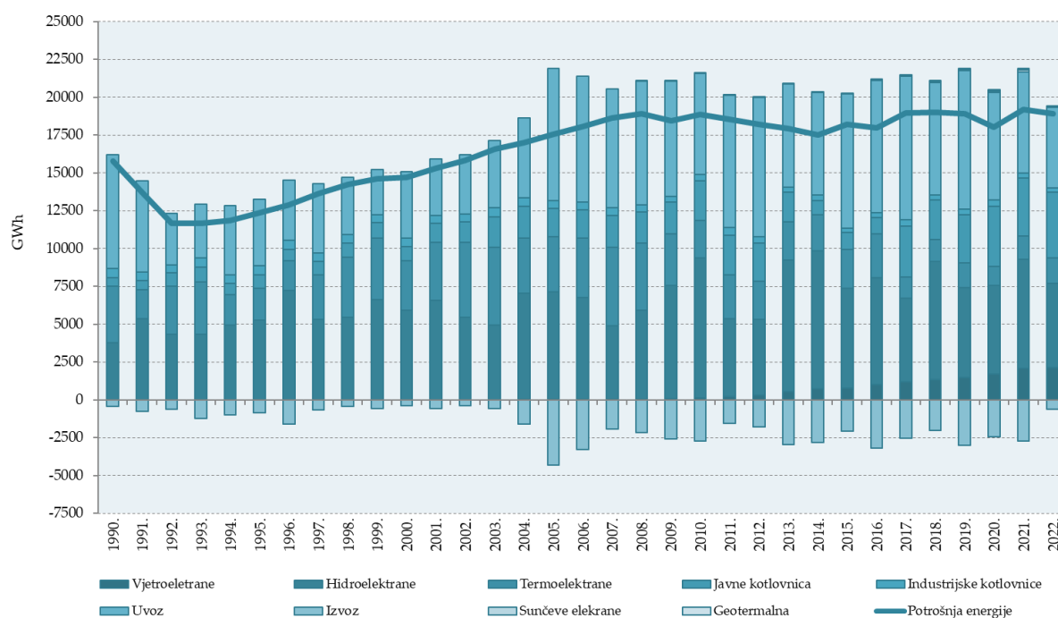
Slika 3.2-2: Potrošnja električne energije za razdoblje od 1990. do 2022. godine
