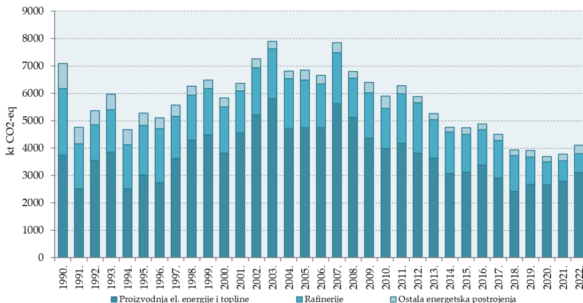
Slika 3.2-1: Emisija CO 2 -eq podsektora Energetskih transformacija
