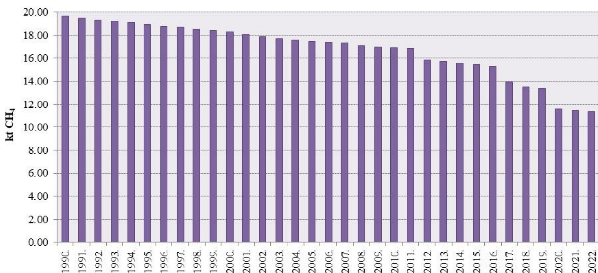
Slika 7.5-1: Emisije CH 4 iz kategorije 5.D.1 Otpadne vode kućanstava (1990. - 2022. godina)
