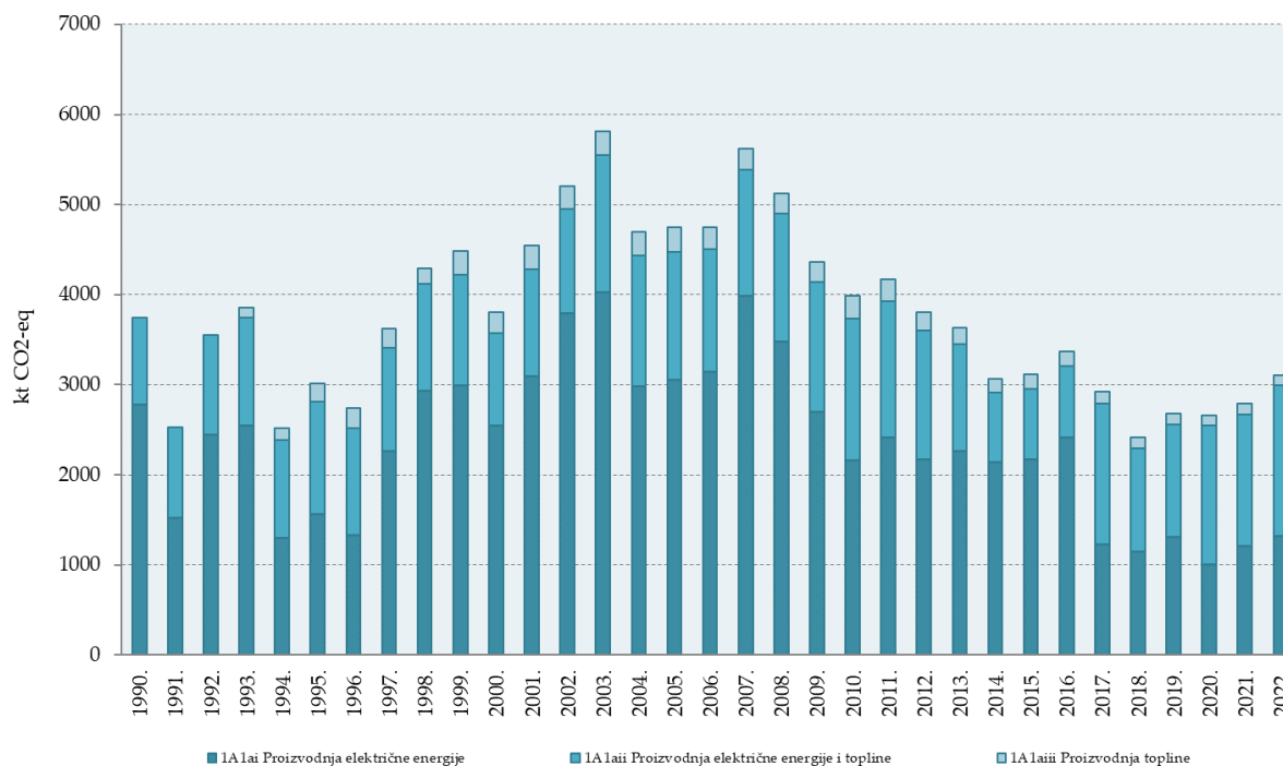
Slika 3.2-3: Emisija CO 2 -eq iz podsektora proizvodnje električne energije i topline
