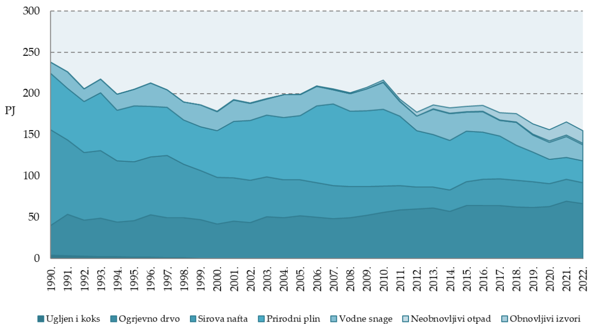
Slika 3.1-1: Trend ukupne proizvodnje primarne energije od 1990. do 2022. godine
