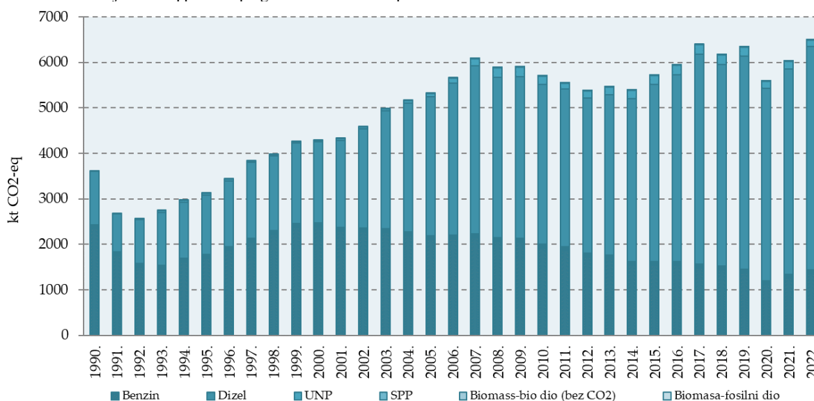
Slika 3.2-9: Emisije CO 2 -eq prema tipu goriva u cestovnom prometu
