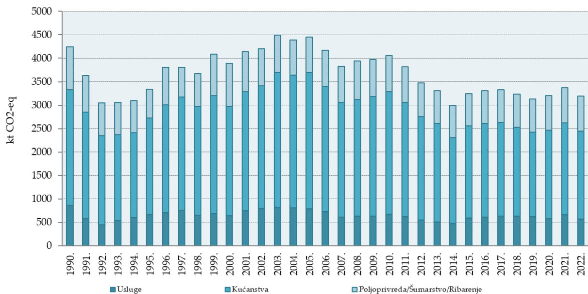
Slika 3.2-12: Emisija CO 2 -eq (kt) podsektora Opće potrošnje
