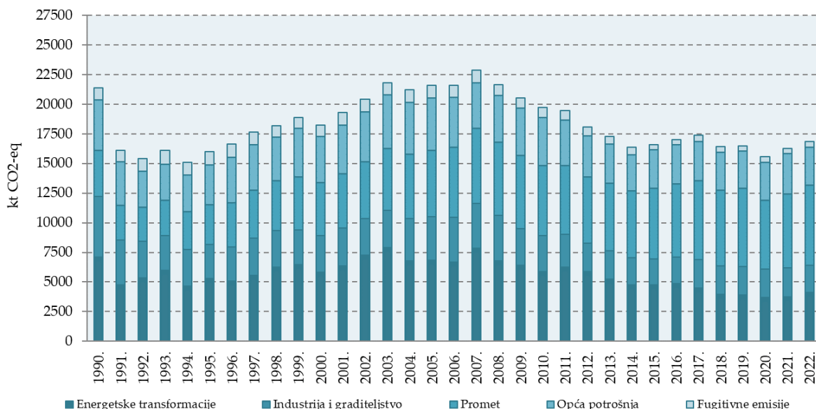
Slika 3.1-6: Emisija CO 2 -eq energetskeg sektora po podsektorima u razdoblju od 1990. do 2022. godine
